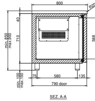
SEZ. A-A
