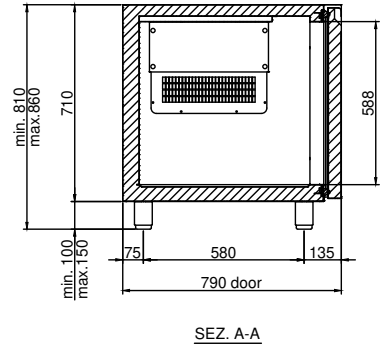
SEZ. A-A
