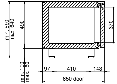
SEZ. A-A
