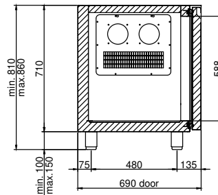
SEZ. A-A
