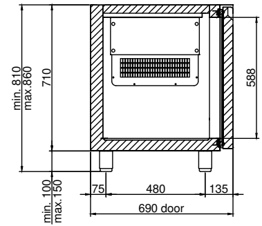
SEZ. A-A
